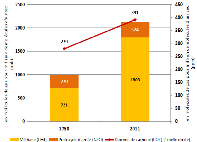
Evolution des concentrations atmosphériques des gaz à effet de serre entre 1750 et 2011
